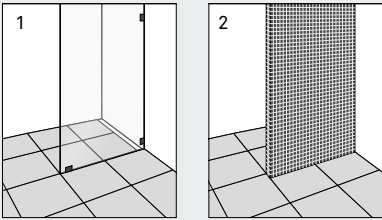
INSTALLATIONSEKSEMPLER 1.ShowerLine med brusevæg 2.ShowerLine med muret væg
